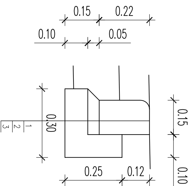
krawężnik na ławie z oporem (zatopiony)
