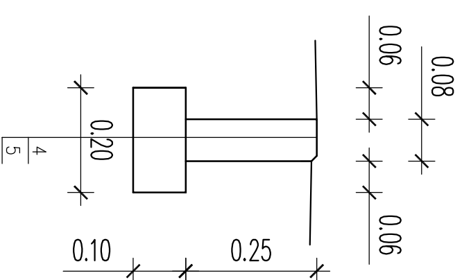
obrzeże na ławie zwykłej
